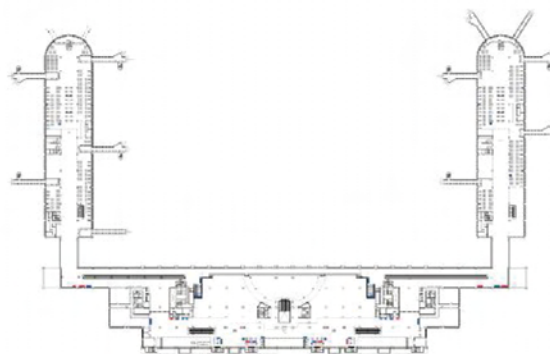
■那覇空港2階平面図
